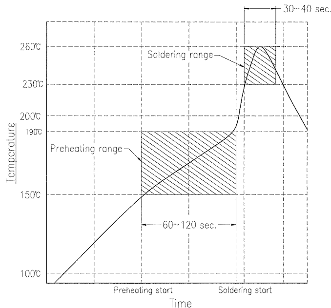
図 2.推奨リフロー温度プロファイル
